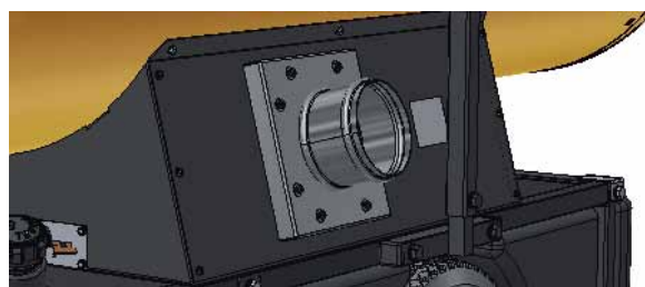
Kit di presa aria secondaria consente di collegare un tubo flessibile di alimentazione aria comburente. Risulta molto utile in caso di aria ambiente inquinata.
