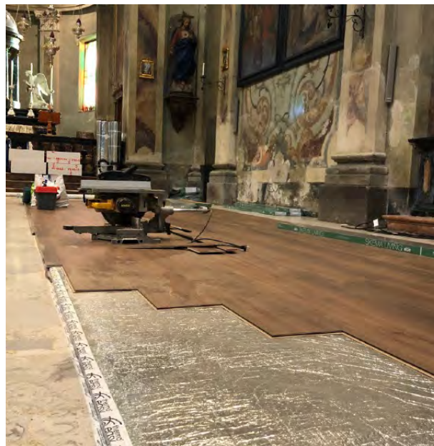
INSTALLAZIONE DEL PAVIMENTO FLOTTANTE SOPRA AL RADIANTE
