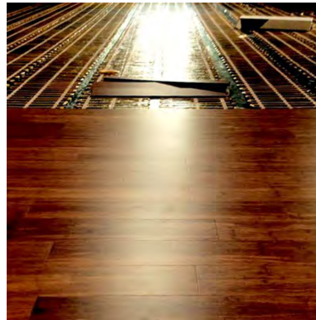
POSA DEL PAVIMENTO FLOTTANTE SOPRA AL RADIANTE
